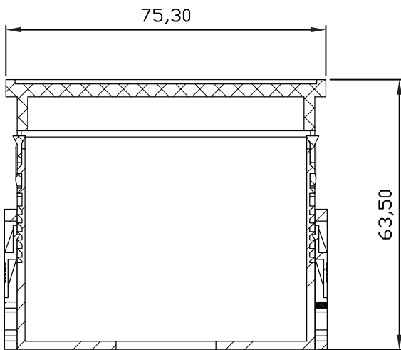
SEÇÃO A-A
